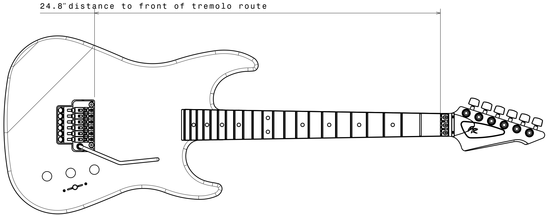
Front view Scale: 1:4
